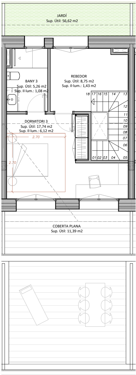
PLANTA SOTACOBERTA
