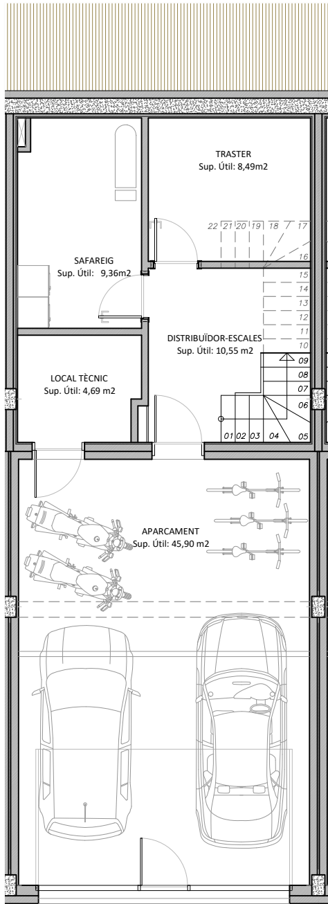
PLANTA SOTERRANI
