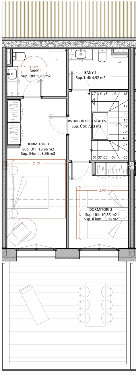
PLANTA PRIMERA
